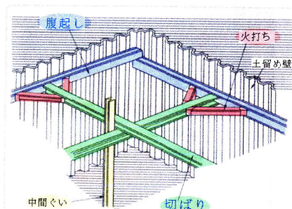
【鋼矢板土留め支保工】
